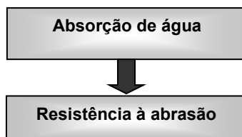
Figura 3 - Exemplo de fluxograma de ensaio de massas niveladoras de empresas não participantes do Programa
