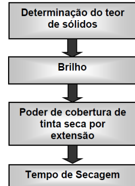
Figura 4 - Exemplo de fluxograma de ensaio de esmaltes sintéticos de empresas não participantes do Programa
