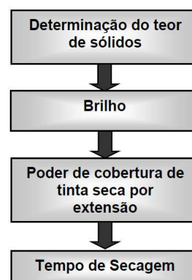
Figura 4 - xemplo de fluxograma de ensaio de esmaltes sintéticos de empresas não participantes do Programa
