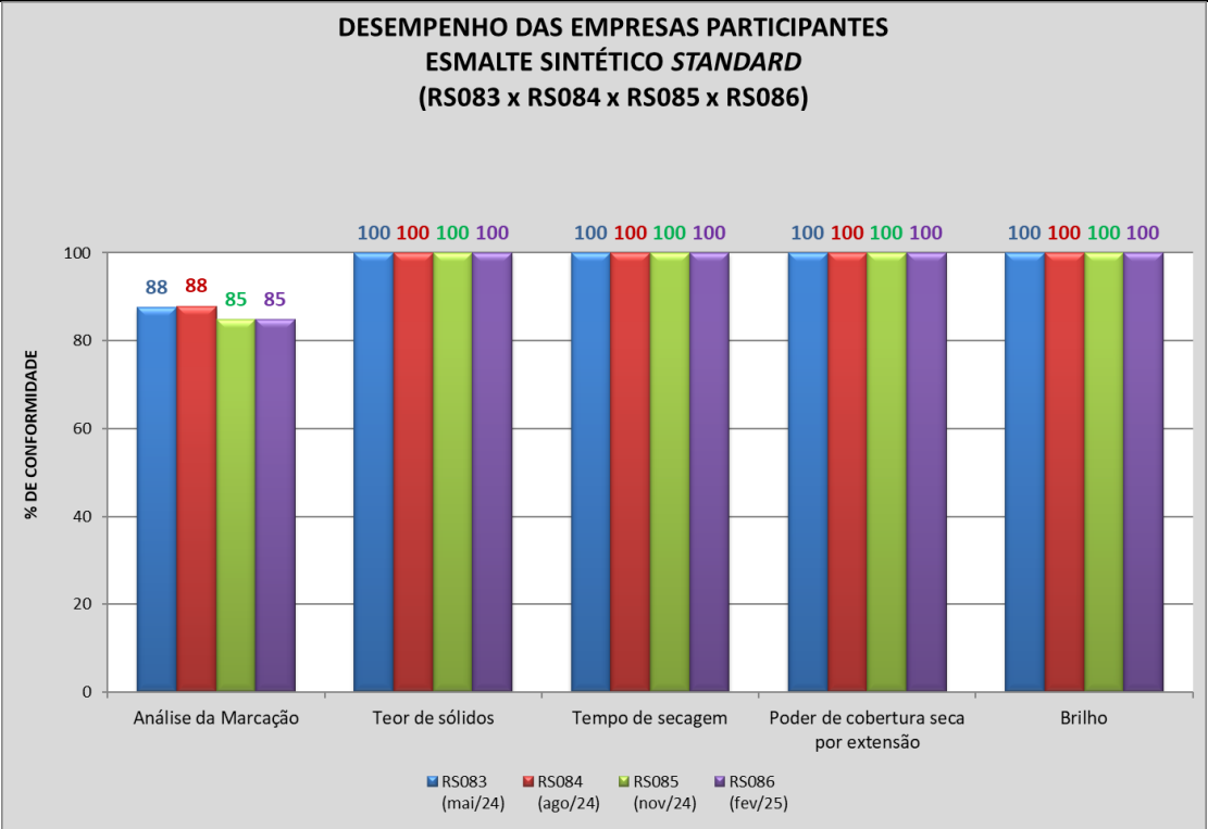
Figura 14 - Evolução das empresas PARTICIPANTES para cada análise de esmalte sintético standard e tinta a óleo realizada no âmbito do Programa de Qualidade
